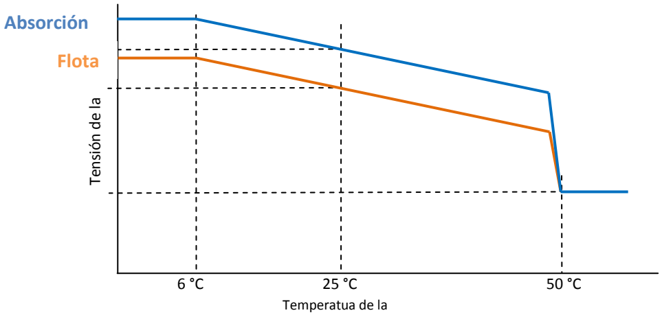
Figura 1: curva de compensación de temperatura
